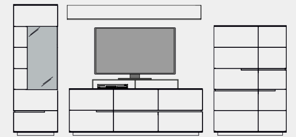
AC-77460 B 368 H 177,4 T 56,1
